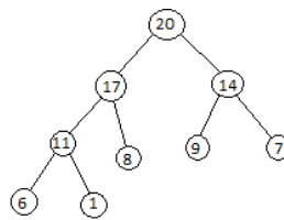
Max-Heap
